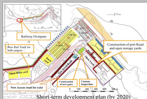
短期整備計画図（出典：ナカラ港開発事業準備調査報告書、JICA、2011年6月）
